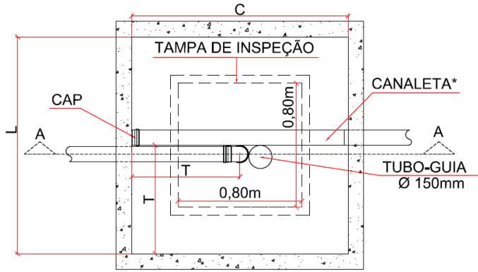
PLANTA BAIXA
