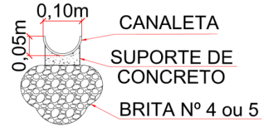
*DETALHE CANALETA
