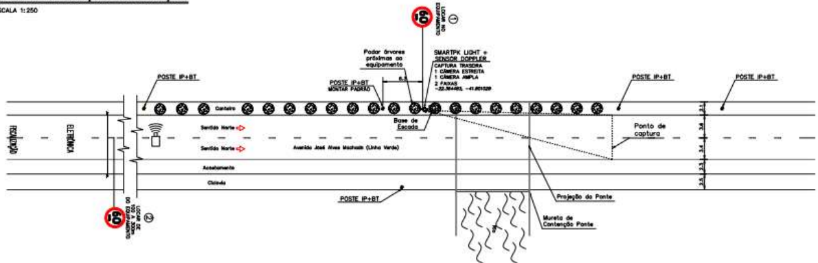
PONTO DE INSTALAÇÃO E SINALIZAÇÃO ESCALA 1:250
