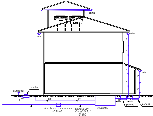
CORTE ESQUEMÁTICO ESC.: 1 : 100 - SISTEMA DE CAPTAÇÃO DE ÁGUAS PLUVIAIS
