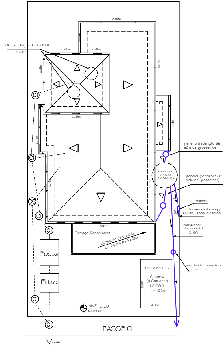
PLANTA DE SITUAÇÃO ESC.: 1 : 100 - ESGOTO E SISTEMA DE CAPTAÇÃO DE ÁGUAS PLUVIAIS
